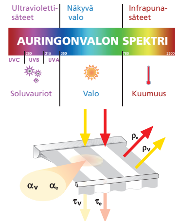
Kuva näyttää symbolit: läpäisy r (Tau), heijastus p (Rho), valon spektrin laskennallisen arvon v, näkyvän valon e eristyksen ja näkyvän valon absorptioon a (alpha). Punainen nuoli kertoo lämpösäteilystä ja keltainen nuoli näkyvästä valosta
